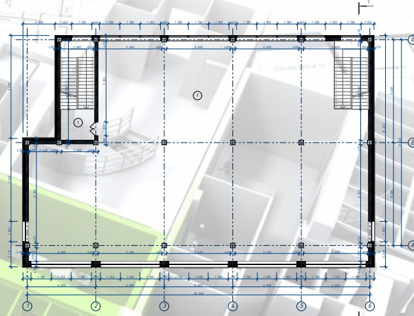
План 2-го этажа на отм. 4,800
