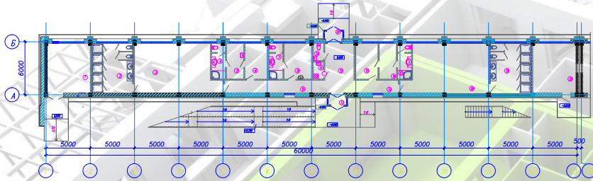
Схема на отм. 0.000
