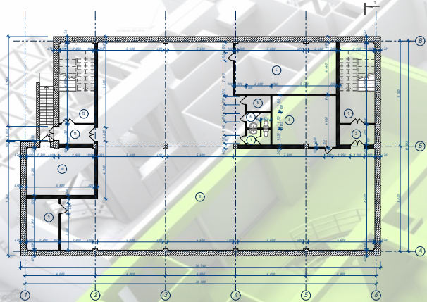
План подвального этажа на отм. -0,000
