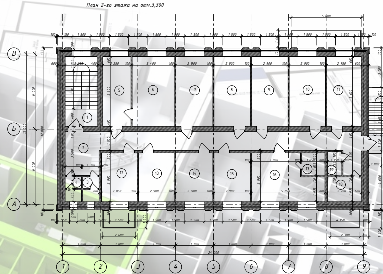
План 2-го этажа на отм.3,300
