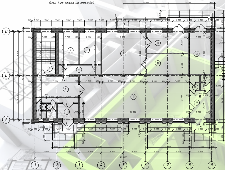
План 1-го этажа на отм.0,000
