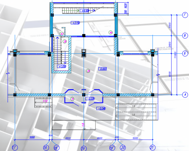
Схема на отм. +3.150
